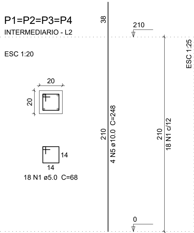
Detalhe Pilares – Caldeira escala →
