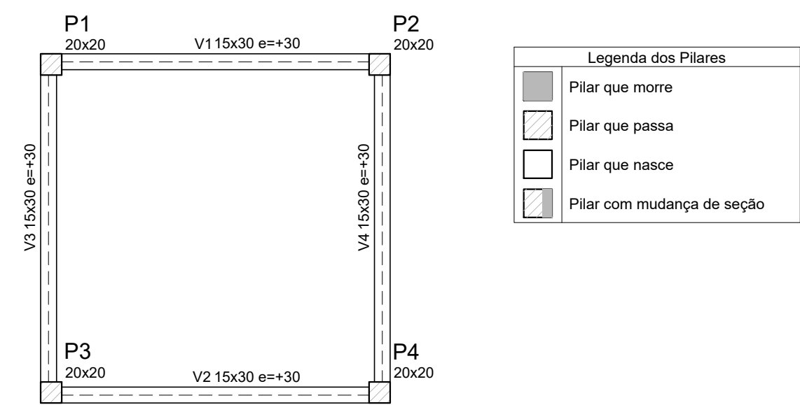
Forma Intermediaria – Caldeira escala → 1/50
